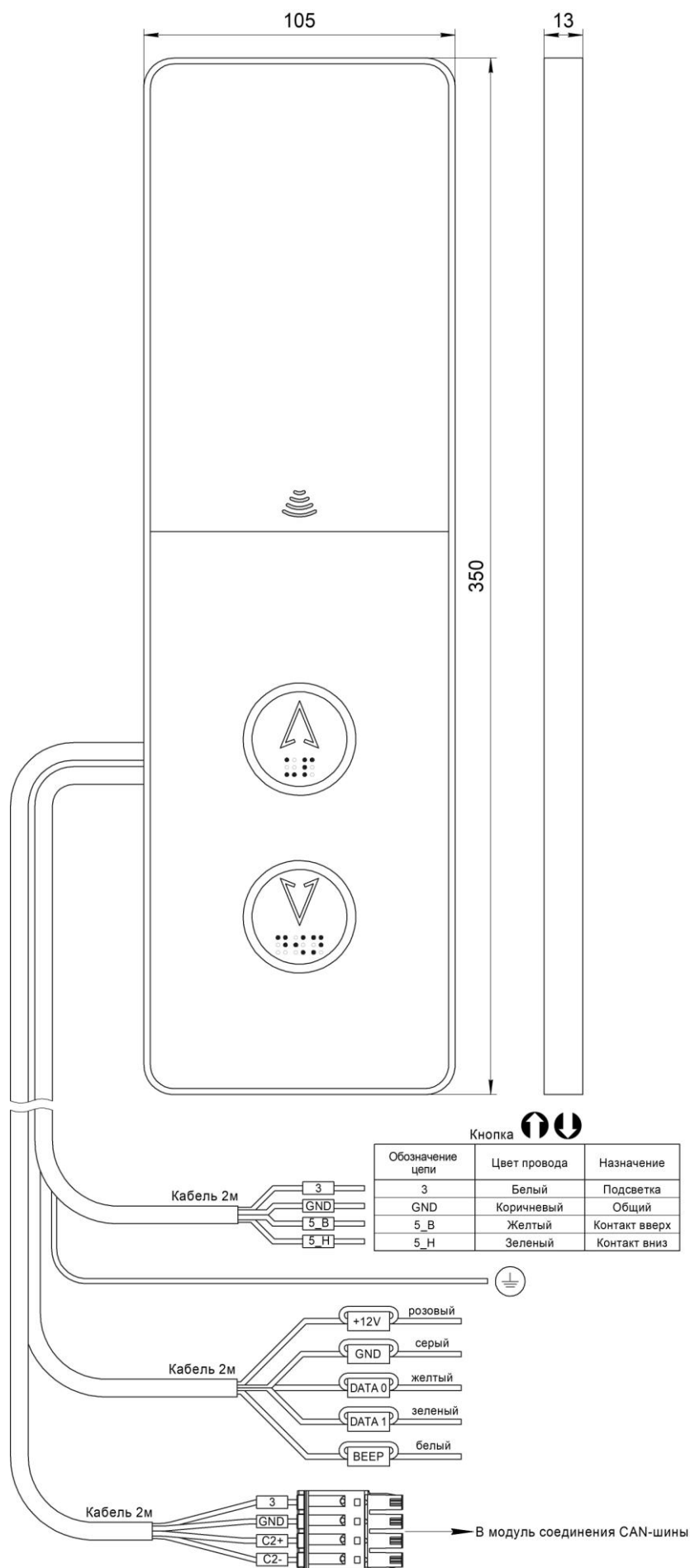
Рис.1 Внешний вид, габаритные и установочные размеры Вызывного поста Малахит НСЕК.468381.016-09
